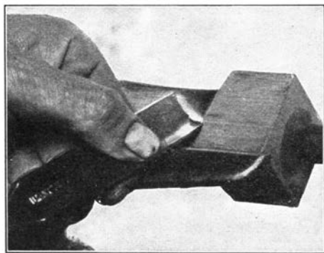
Fig. 78. Rolling Gouge.
