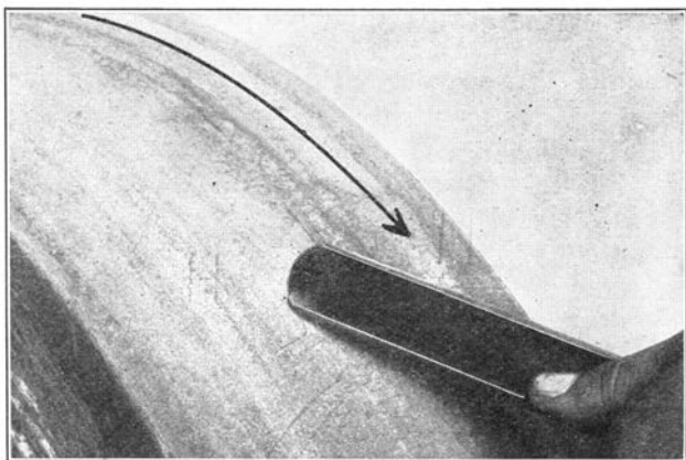
Fig. 284. Grinding a Gouge.
