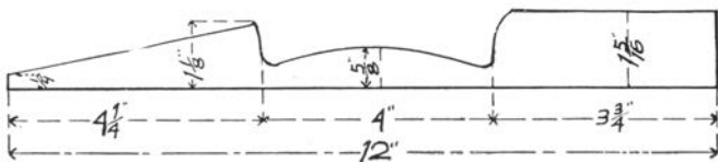
Fig. 155. Molder's Rammer.
