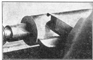
Fig. 16. Using a Skew Chisel.
