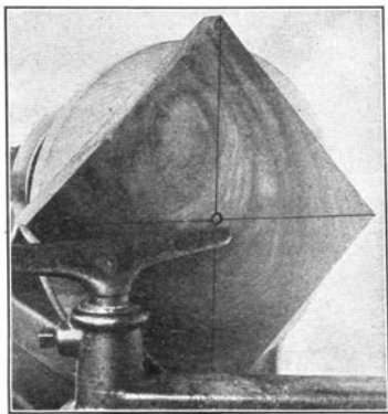
Fig. 230. Frame Blank on Face-plate.
